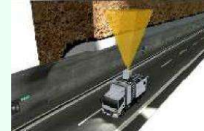
DXを活用したトンネル点検
