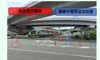
車線分離標等の改善
