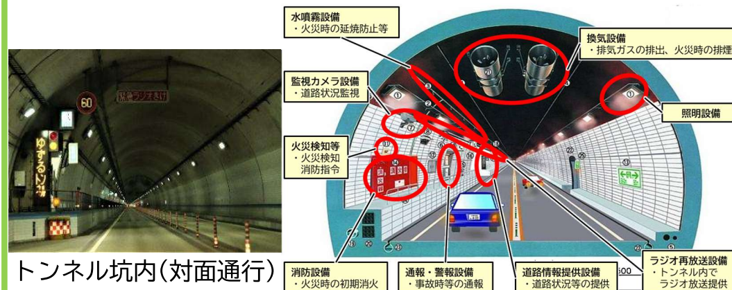
トンネル設備概要
