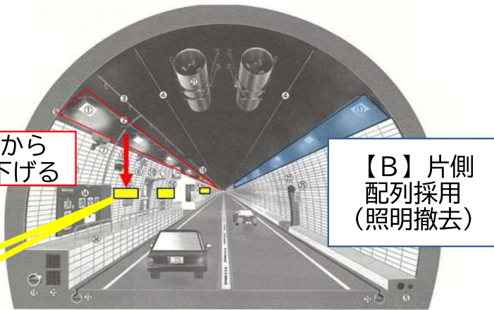
トンネル照明設置の見直し案
